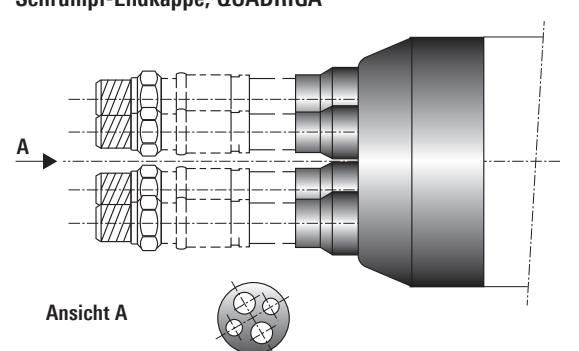
Schrumpf-Endkappe, QUADRIGA
