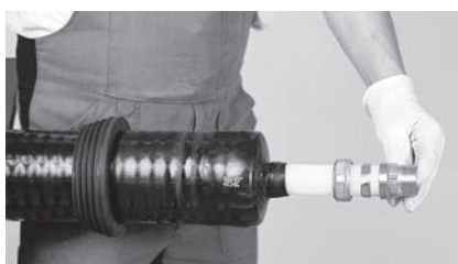
8 Fitting montieren gemäss beigefügten Montageanleitungen.
